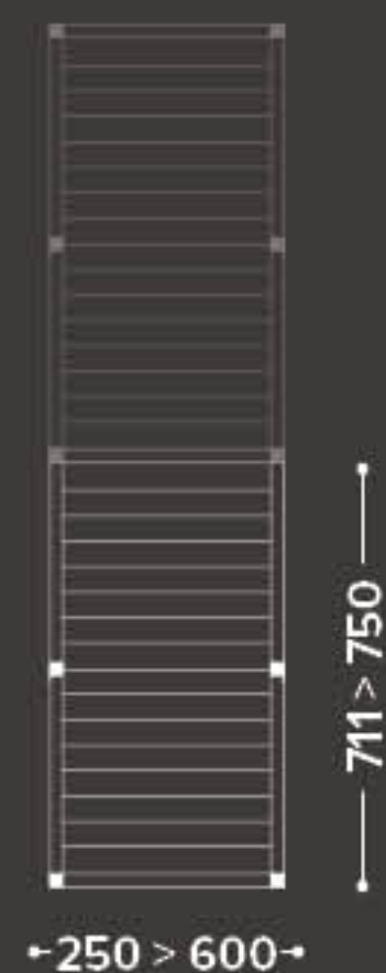
ISOLA / ISLAND modulo accoppiato 4 gambe coupled module 4 posts
