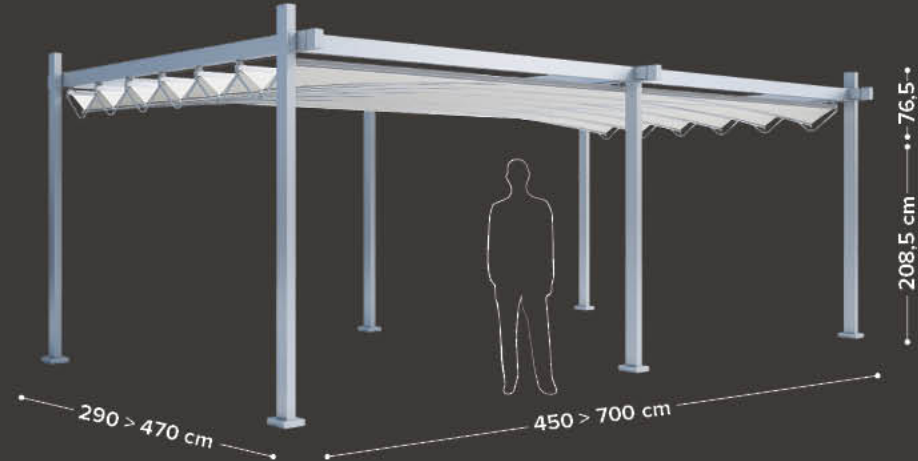
ISOLA / ISLAND doppio modulo 6 gambe coupled module 6 posts
