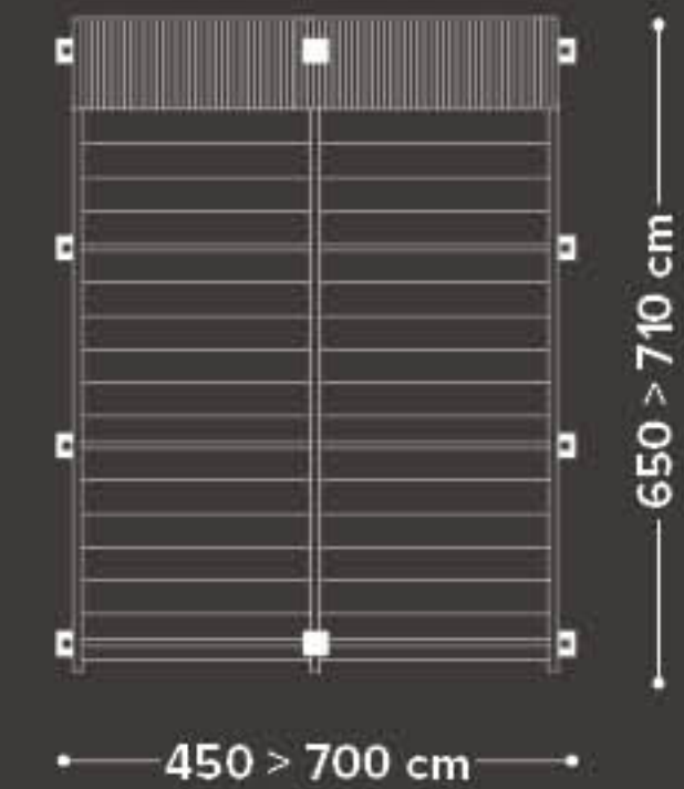
ISOLA / ISLAND doppio modulo 10 gambe coupled module 10 posts
