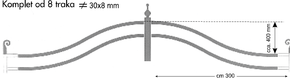
Art. BL 257 Komplet od 8 traka ≠ 30x8 mm
